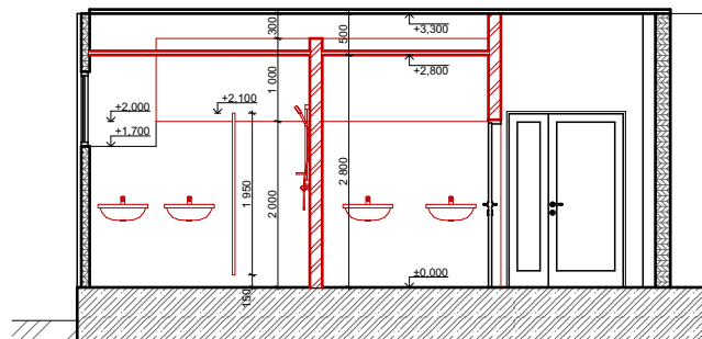
Rez A-A - nový stav
