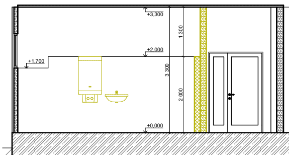
Rez A-A - pôvodný stav
